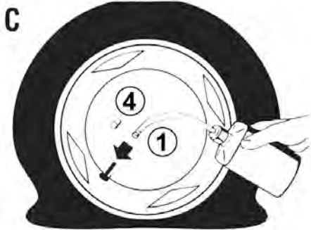
Einfüllschlauch auf Reifenventil aufschieben
