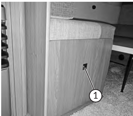
Pushlock-Sicherung
