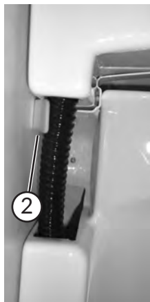
Mechanismus Klappwaschbecken
