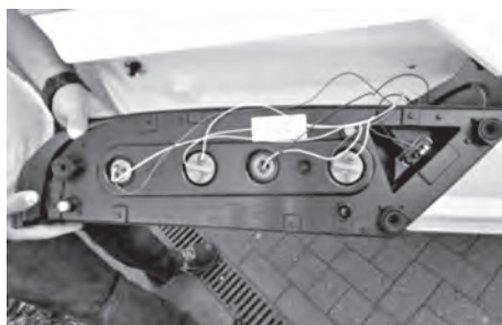
Rücklicht Rückseite
